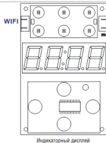
Индикаторный дисплей
